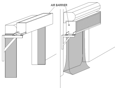
Roll Up Door (RU)
